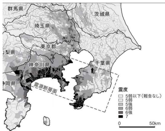
関東地震の推定震度分布
