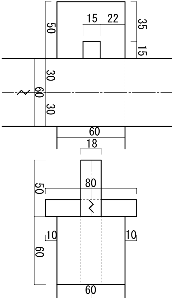
束柱・頭繋ぎ取り合い部詳細
