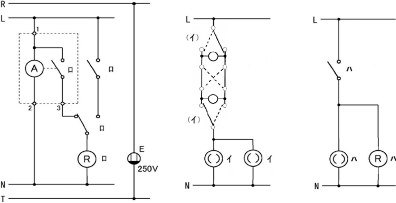
【展開接続図】
