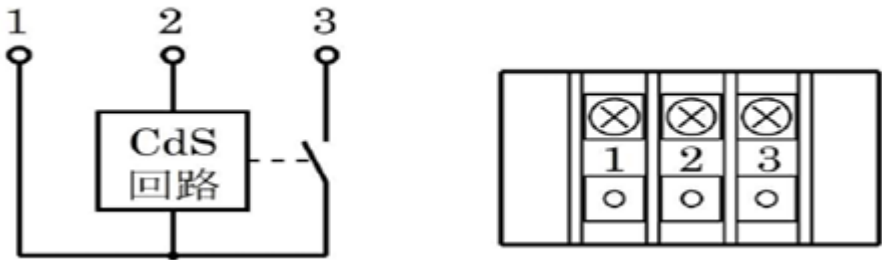
内部結線図
