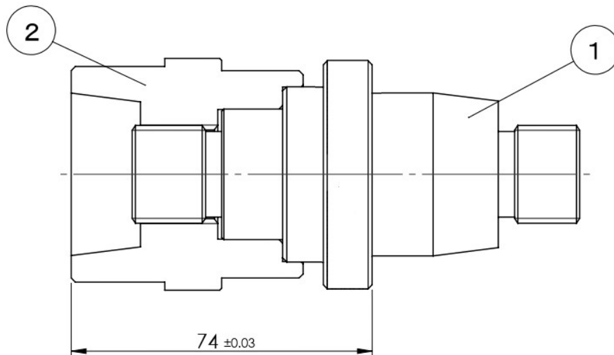
組立図B
