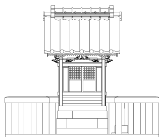
観蓮寺稲荷社 正面図
