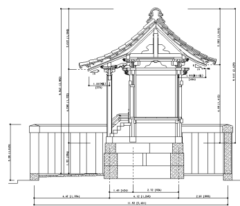
観蓮寺稲荷社 梁間断面図
