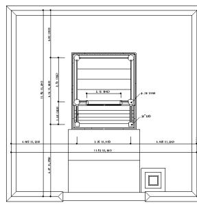
観蓮寺稲荷社 平面図
