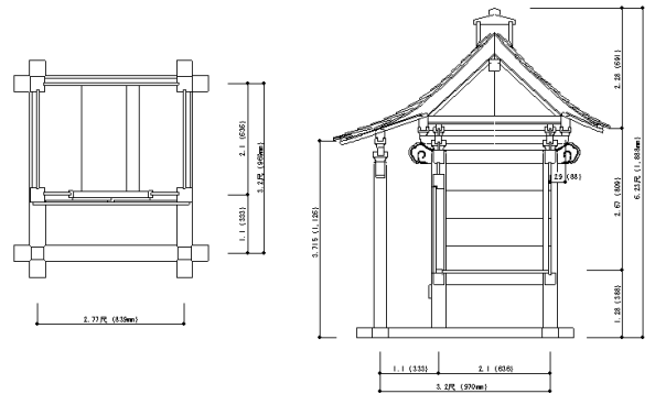
城本八幡皇神社 平面図・梁断面図
