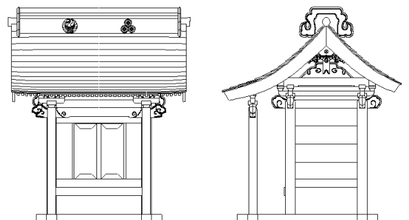
城本八幡皇神社 正面図・側面図
