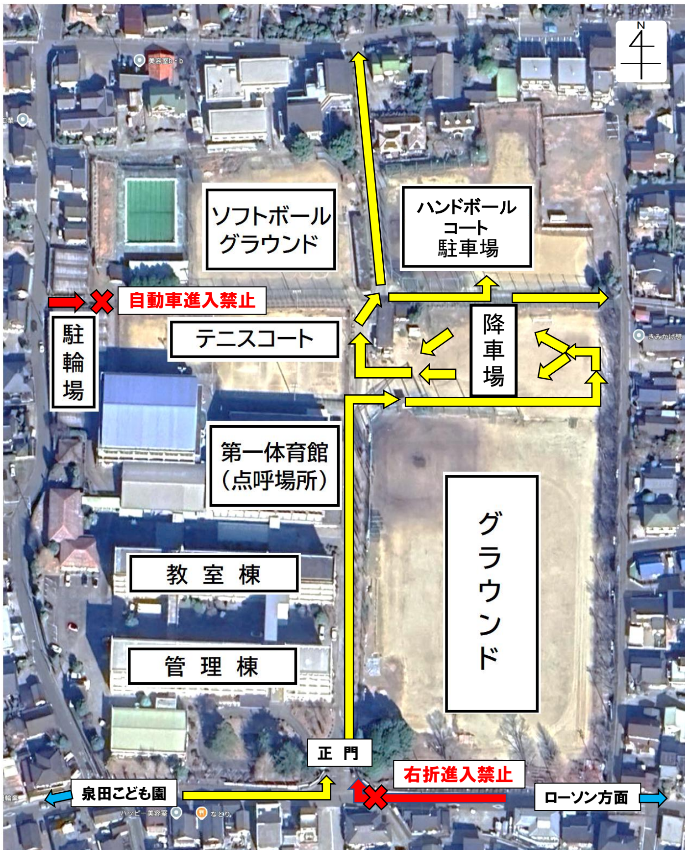
周辺地図
